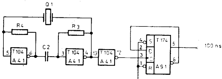
Abb. 6 Taktgenerator
