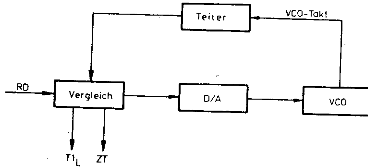
Abb. 8 Blockschaltbild PLL-Schaltung
