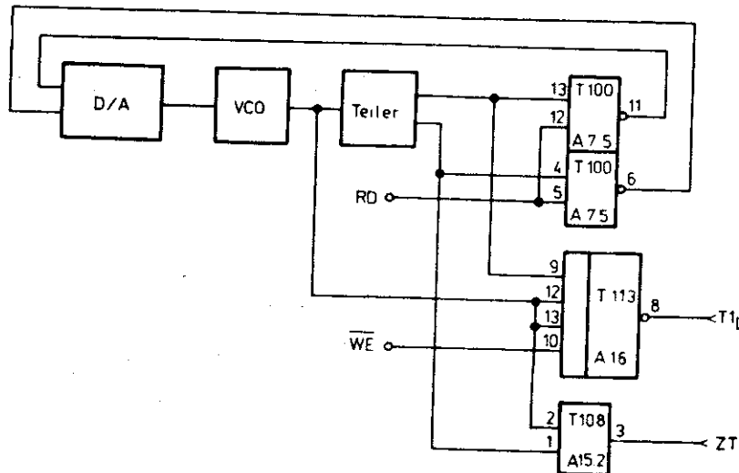
Abb. 9 Taktbildung Lesen
