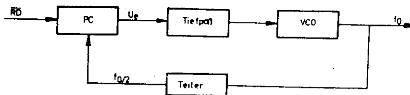
Abb. 1 Blockschaltbild
