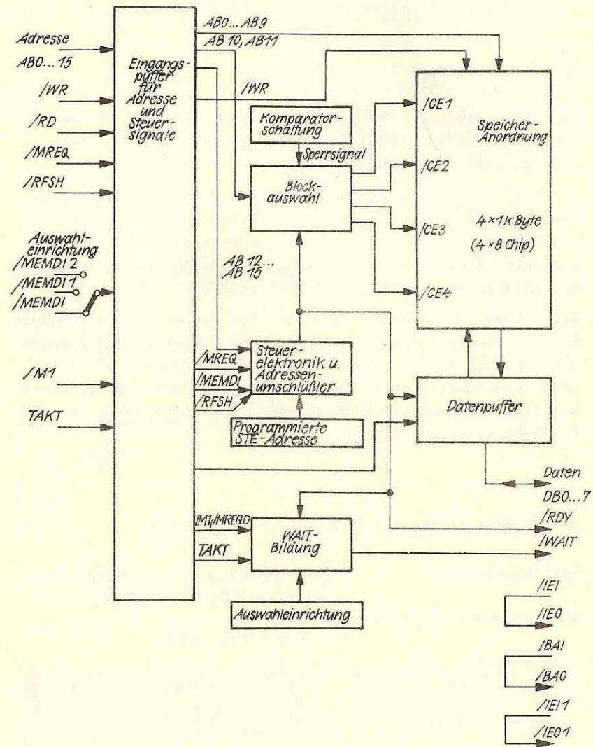
Abb. 2 Blockschaltbild K 3520
