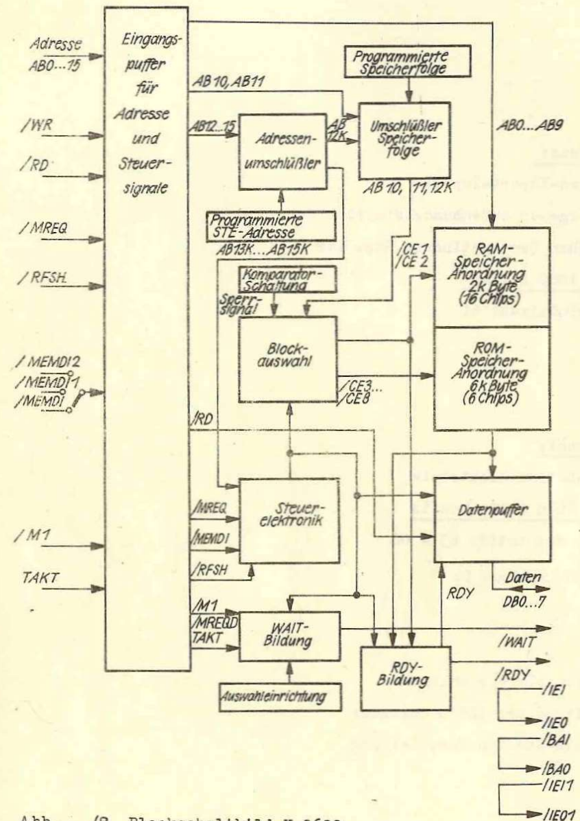
Abb. /8 Blockschaltbild K 3620
