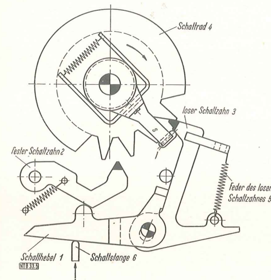
Bild 5. Schrittschaltwerk der Rheinmetall-Schreibmaschine Schaltrad: Durchmesser D = 36 mm Zähnezahl z = 18 Übersetzung: i = \frac{s_{\text{Wagen}}}{s_{\text{Schaltr.}}} = \frac{2,6}{6,28} = 0,414; i = 0,414:1
