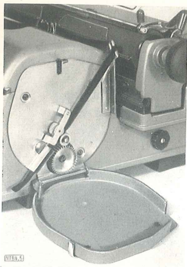
Bild 5. Kohlebandeinrichtung für elektrische Schreibmaschinen
