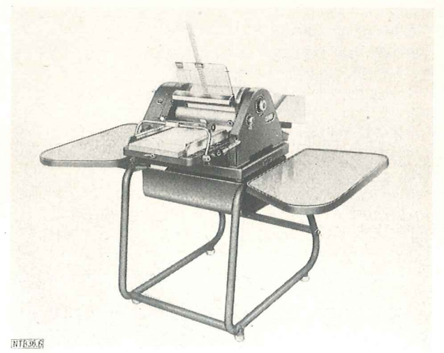
Bild 6. Umdruckvervielfältiger CENTO 240 mit elektrischem Antrieb
