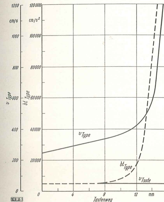
Bild 1. Beschleunigungskurven vom Comбина-Antrieb für den Mittelhebel Nr. 24 (mit Segmentenschaltung); Bewegungsverhältnisse bei v_{T0} = 50 cm/s
