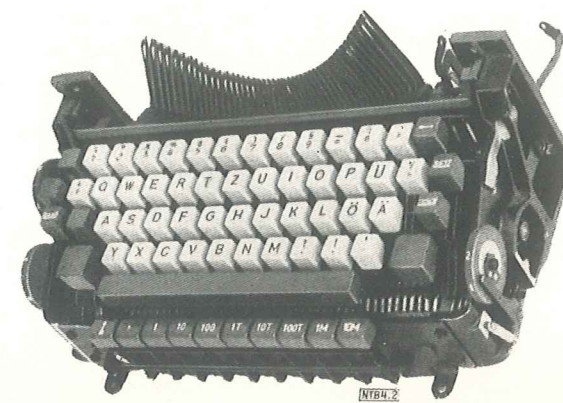
Bild 2. Montageeinheit der Rheinmetall Modell GSE
