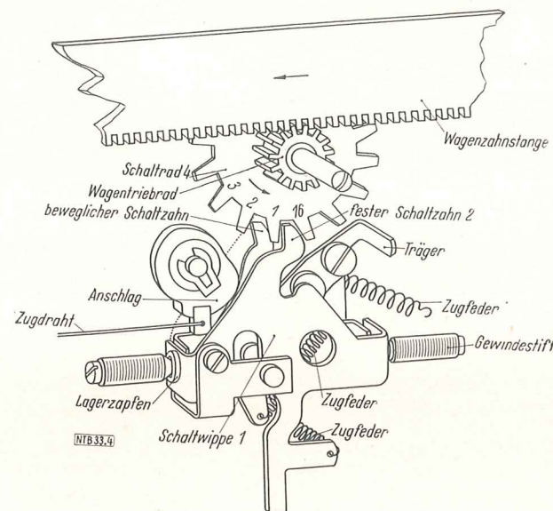
Bild 4. Zusammenwirken von Schaltrad, losem Schaltzahn und Wagen [1]
