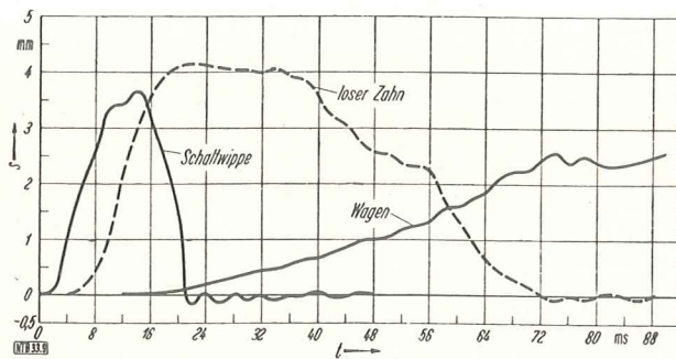
Bild 9. Zusammenwirken von Wippe, Wagen und Schaltzahn
