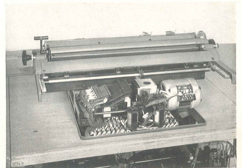
Bild 7. Steuereinrichtungen im rückseitigen Schreibmaschinenteil der Fakturiermaschine
