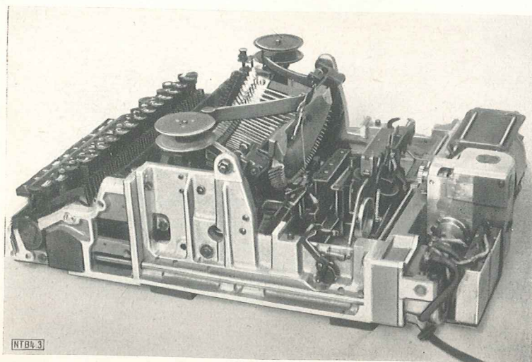
Bild 3. Gesamtaufbau der elektrischen Rheinmetall-Großschreibmaschine ohne Verkleidungshaube
