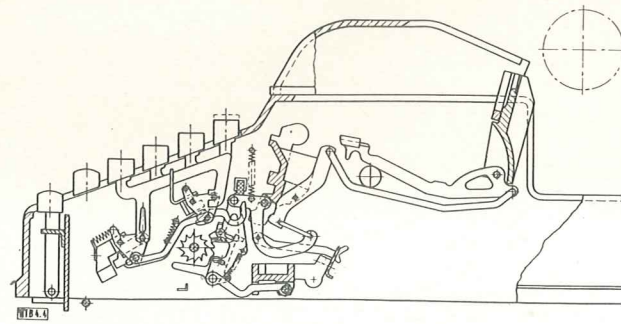
Bild 4. Typenhebelantrieb der „Rheinmetall GSE“ (schematisch)
