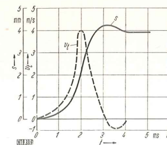
Bild 6. Bewegungsverlauf des losen Schaltzahnes bei einfacher Schrittschaltung
