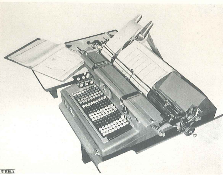
Bild 9. LOG ABAX Buchungs- und Statistikmaschine, Modell „SENIOR“ mit beweglichem Wagen für Horizontal- und Vertikalarbeiten
