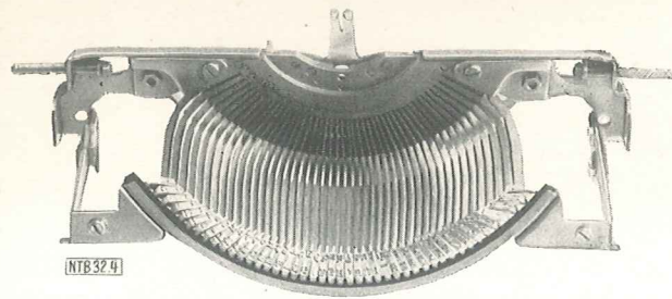
Bild 4. Typenhebellager im Stahlrahmen
