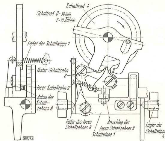
Bild 3. Schrittschaltwerk der Ideal-Schreibmaschine
