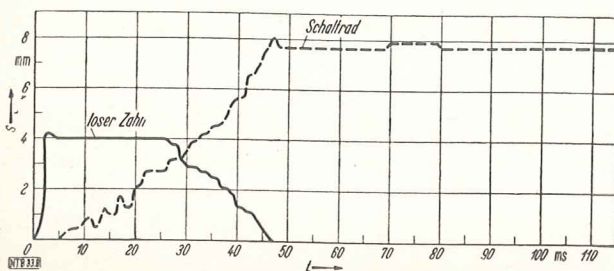
Bild 8. Bewegungsverlauf des Schaltrades
