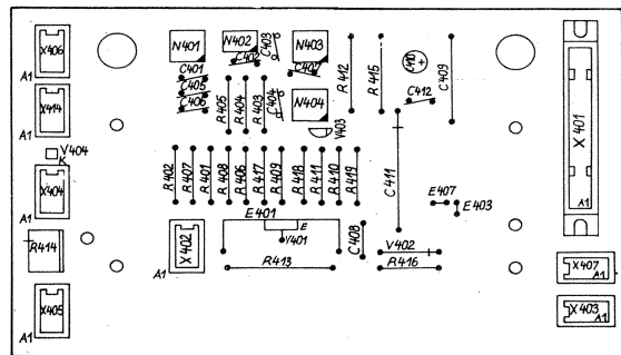
BLP-Druckwagen
